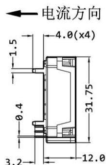
PCB示意图
