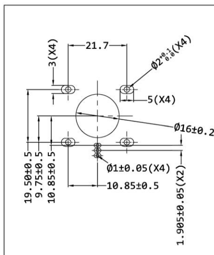
PCB示意图
